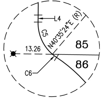
DETAIL 'B' SCALE: 1" = 20'
